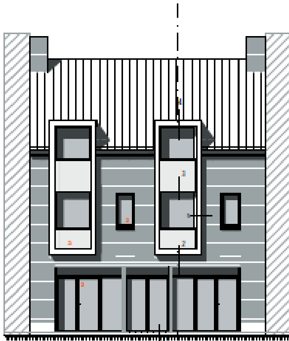
VOORGEVEL Klifweg 9 NIEUW
